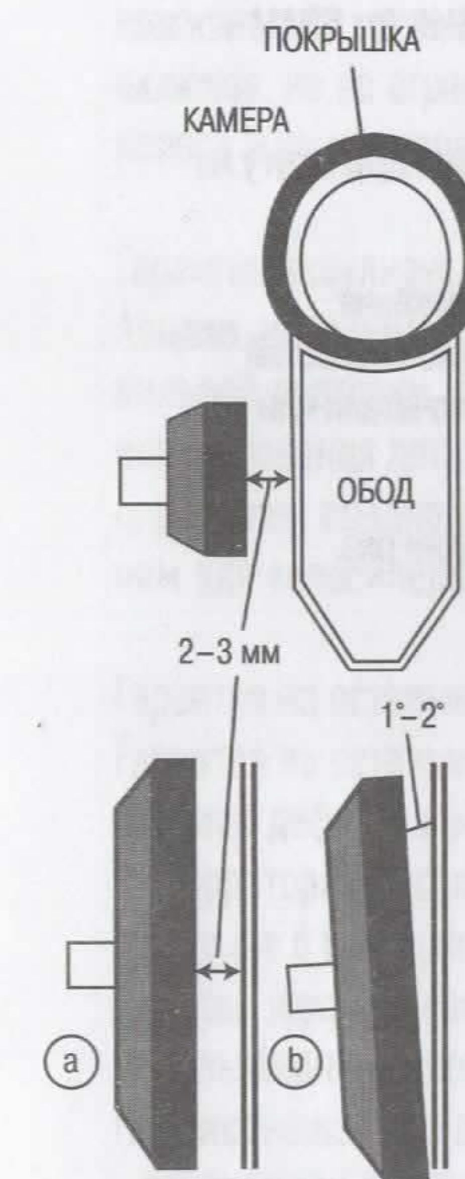
Рис. 9. Установка колодок
