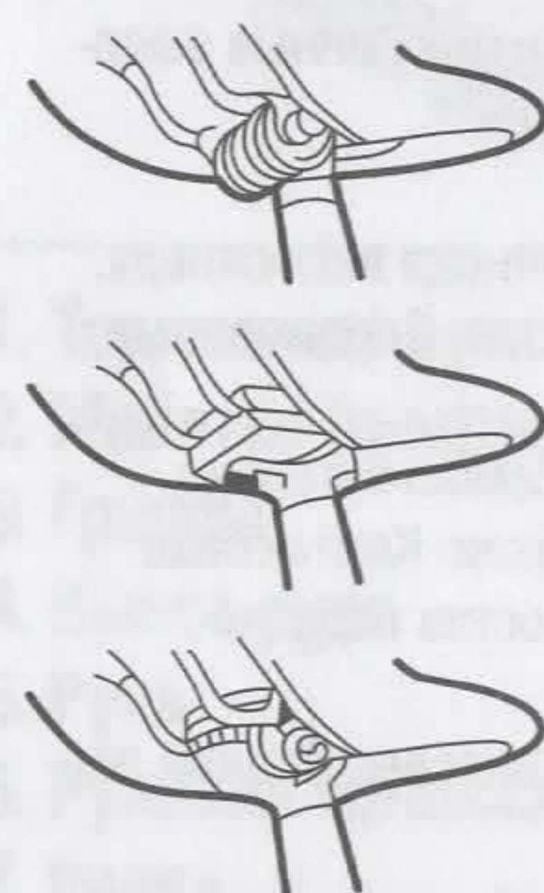
Рис. 2. Тип крепления седла
