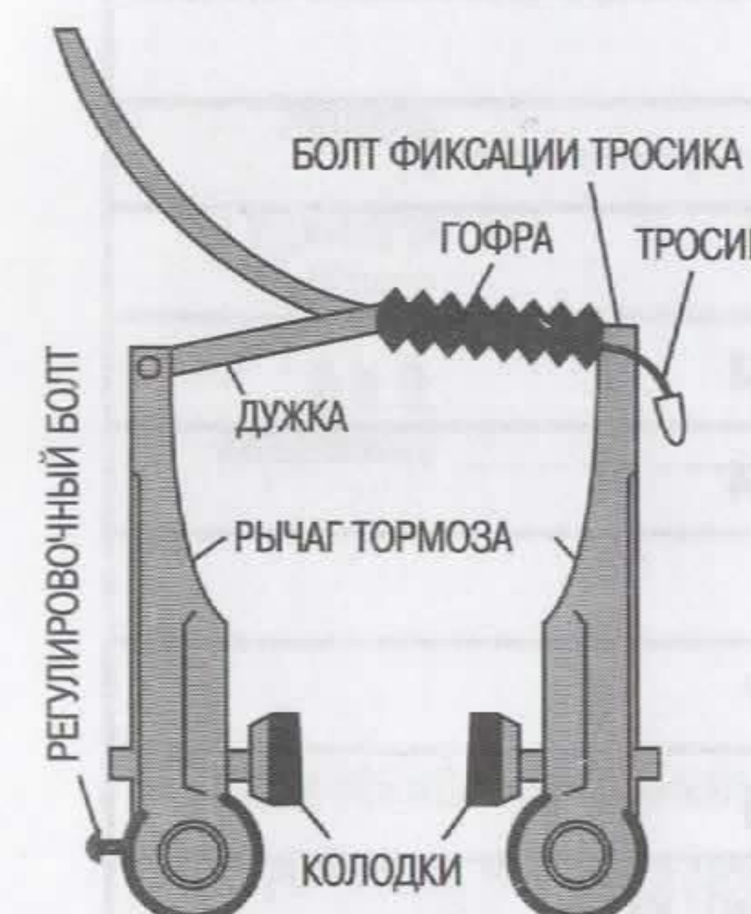
Рис. 8. Общий вид тормоза типа V-Brake
