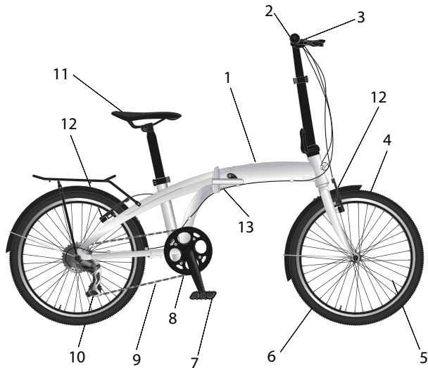
Схема складного велосипеда
